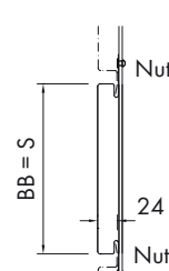
Paneeltyp „D“
