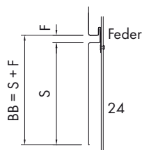
Paneeltyp „B“
