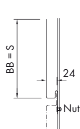
Paneeltyp „C“
