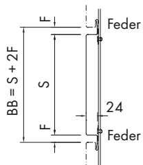
Paneeltyp „A“
